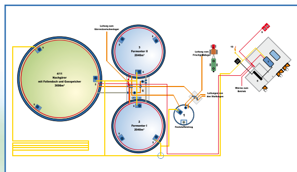
Abb. Fließschema Hohen Wangelin
